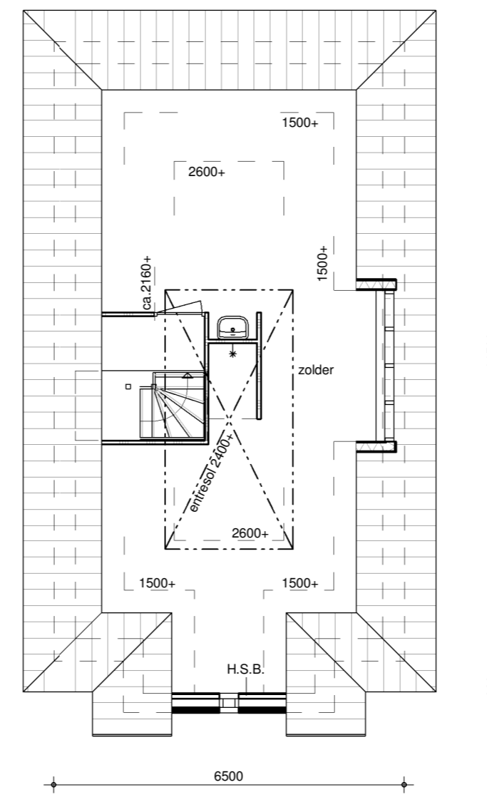
tweede verdieping
